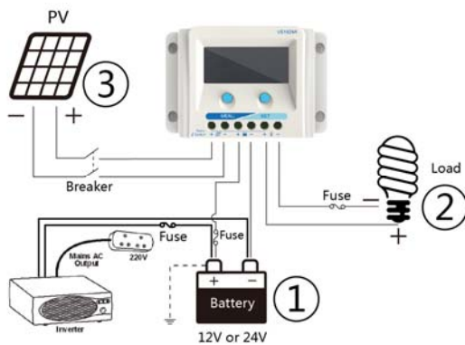
Abbildung 3 Anschlussdiagramm
